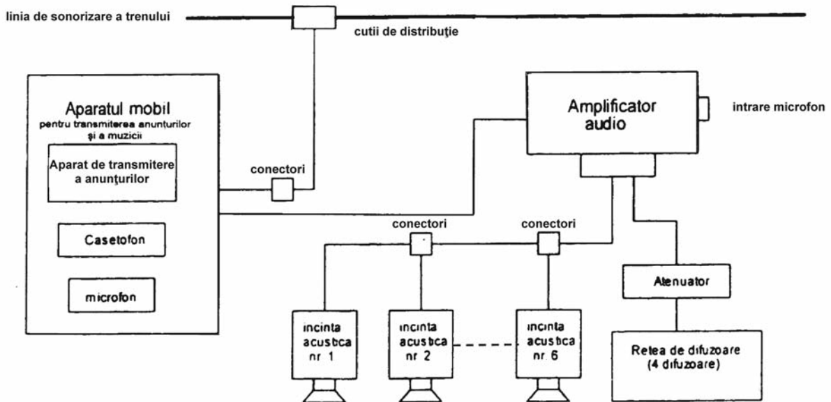
Figura 2 — Exemplu de schemă-bloc a instalației de sonorizare pentru vagoane de clasa a II-a seria 2076
